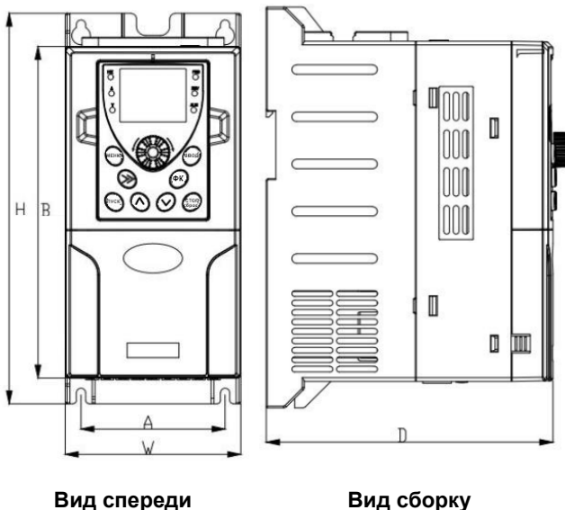
Рисунок 2-1. Габаритные и монтажные размеры преобразователя частоты.
