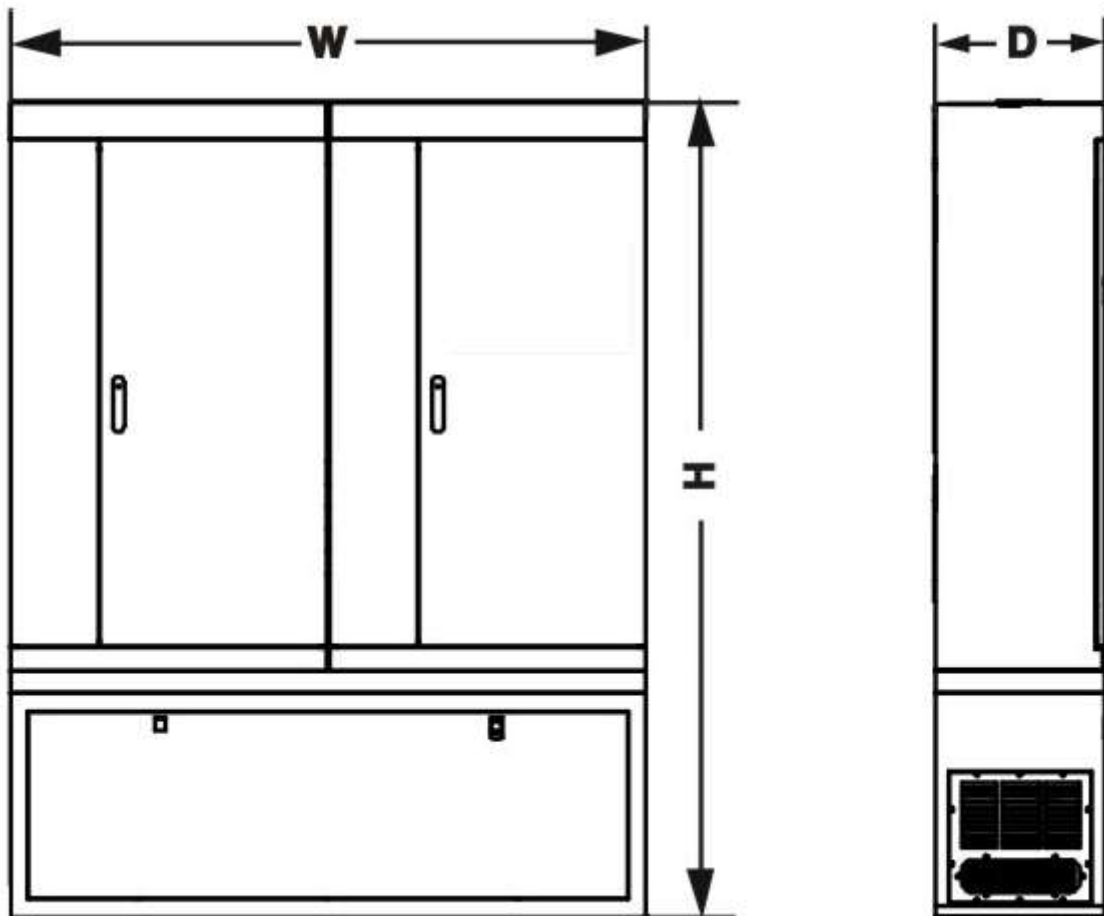
Рисунок А. 4. Габаритные размеры (350–500 кВт)
