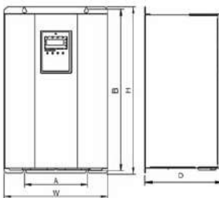
Рисунок А. 6. Габаритные размеры (11–18,5 кВт)
