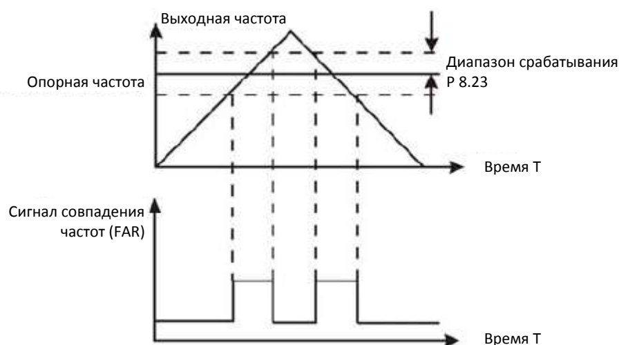
Рисунок 6.22. График сигнала совпадения частот (FAR).
