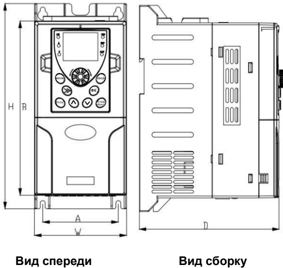
Рисунок 2-2. Габаритные и монтажные размеры преобразователя частоты.
