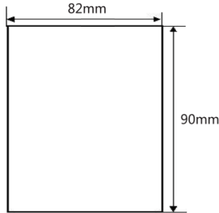
Рисунок 2-3. Размеры монтажного отверстия для установки монтажной рамки.
